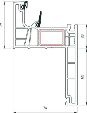
Telaio a ZETA 65 mm
