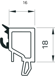
Spessore vetro 38-40mm taglio fermavetro 90°
