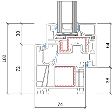
Sistema doppio vetro
