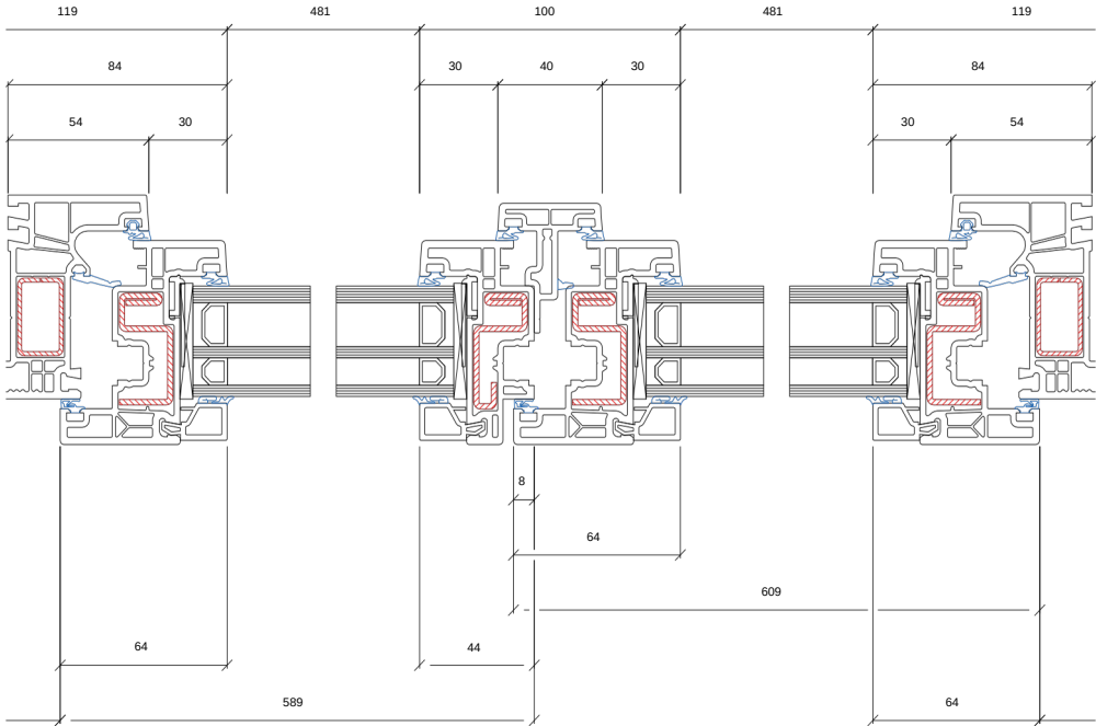
Sezione con Anta Minimal
