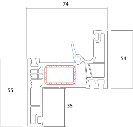
Telaio a ZETA 35 mm
