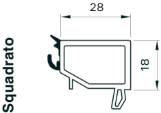
Spessore vetro 28-29mm taglio fermavetro 90°
