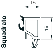
Spessore vetro 38-40mm taglio fermavetro 90°
