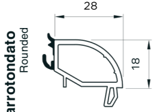
Spessore vetro 28-29mm taglio fermavetro 45°
