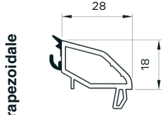
Spessore vetro 28-29mm taglio fermavetro 45°
