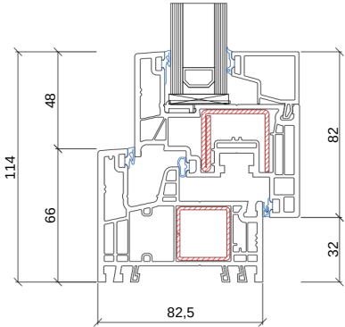
Sistema doppio vetro
