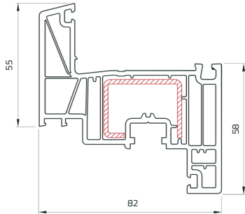
Anta Portoncino Ap. Interna
