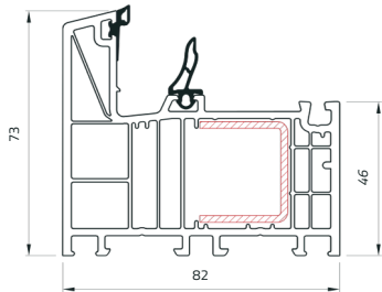
Telaio piano
