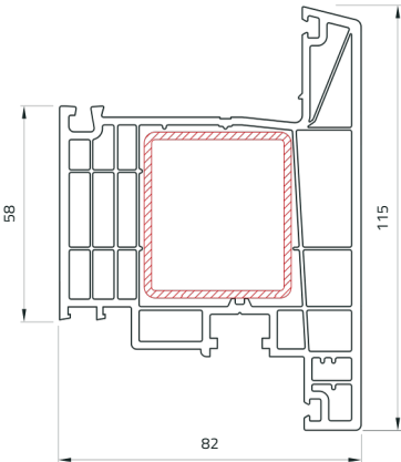
Anta Portoncino Ap. Esterna
