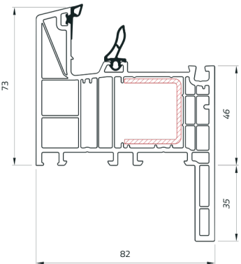
Telaio a ZETA 35 mm
