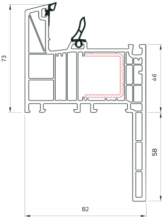
Telaio a ZETA 60 mm
