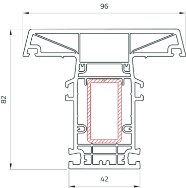
Traverso Montante
