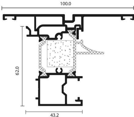
Riporto Centrale Central Carryover
