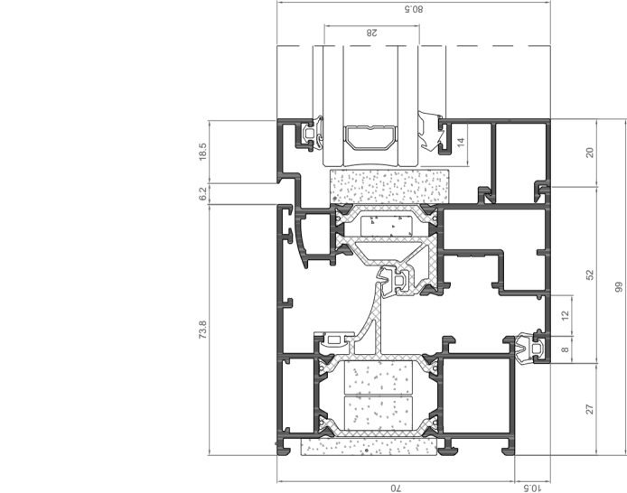
Sistema sezione laterale Double glass system
