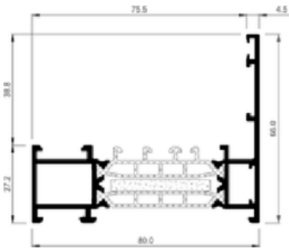
Telaio ad L
