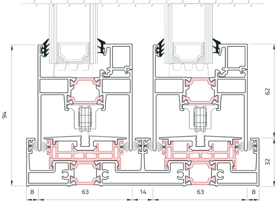
Sistema doppio binario Double tracksystem
