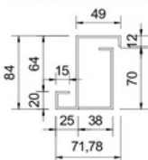
SEZIONE TELAIO E CONTRO TELAIO
